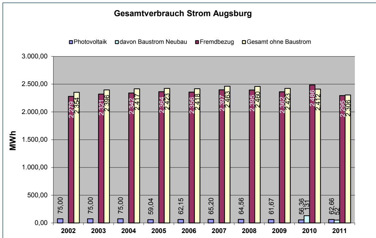
Abb. 2: Gesamtverbrauch Strom
