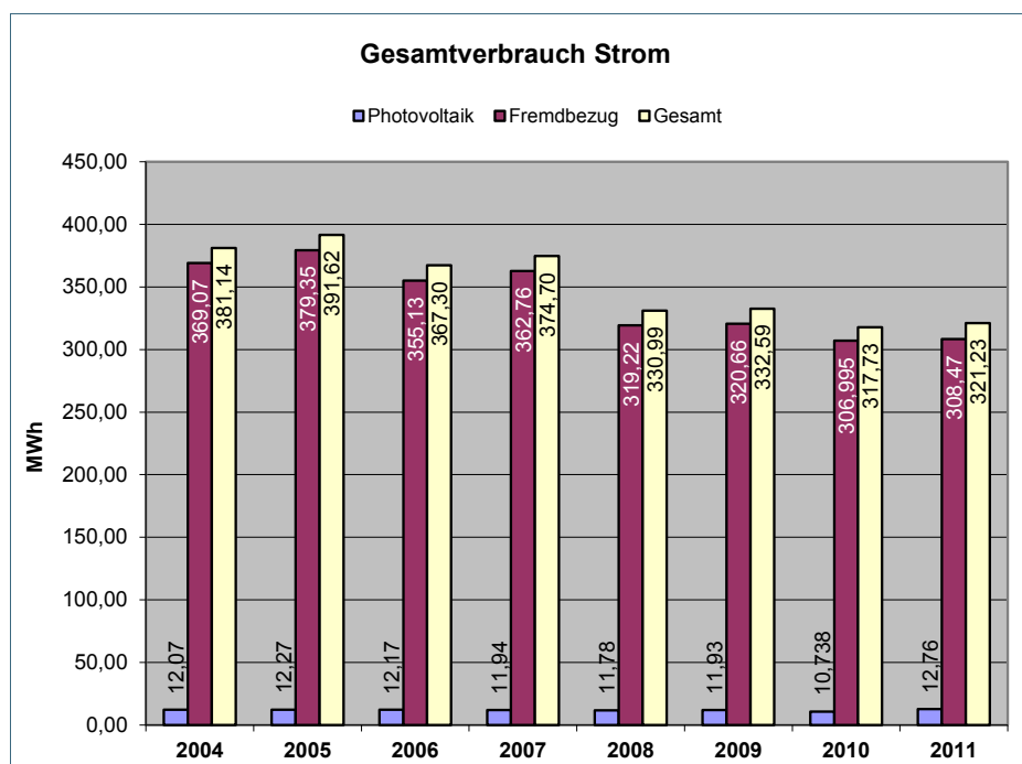
Abb. 26: Stromverbrauch Kulmbach
