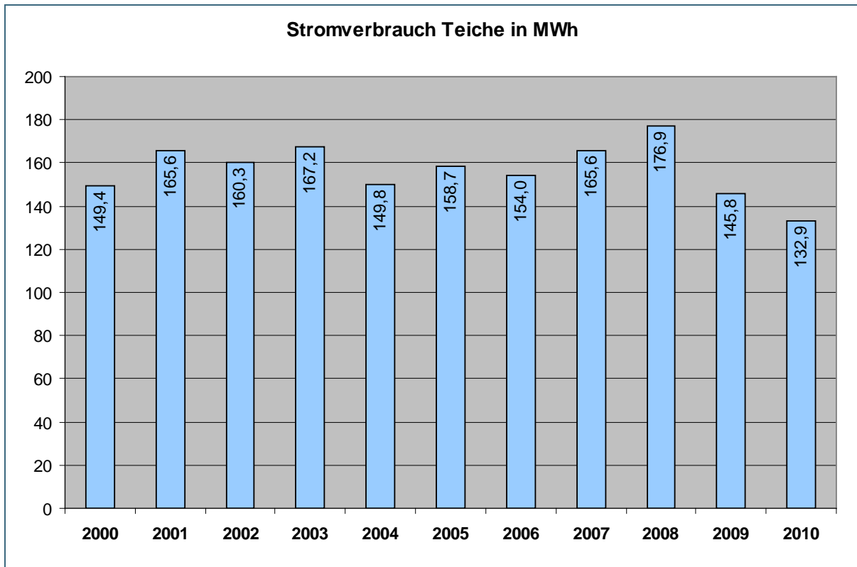
Abb. 47: Stromverbrauch Teiche
