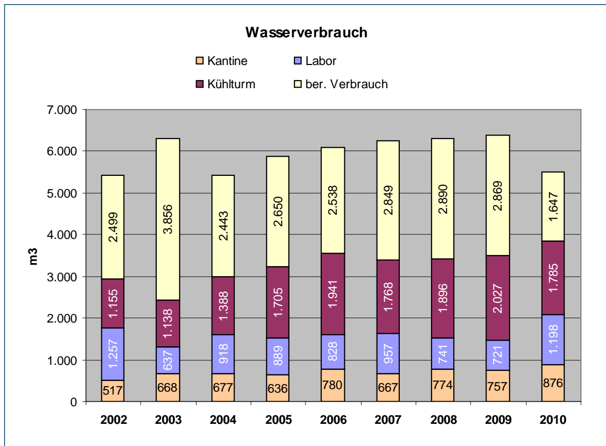
Abb. 26: Wasserverbrauch absolut
