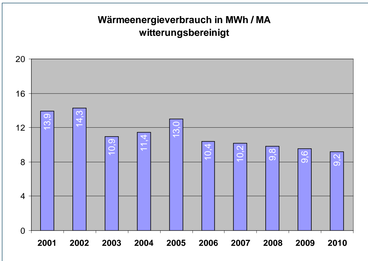
Abb. 52: Witterungsbereinigter Verbrauch pro Mitarbeiter in MWh
