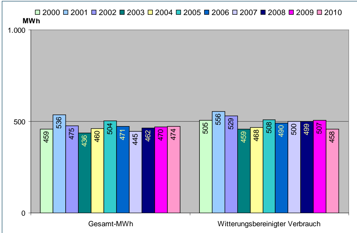
Abb. 51: Verbrauch Wärmeenergie in MWh gesamt und witterungsbereinigt
