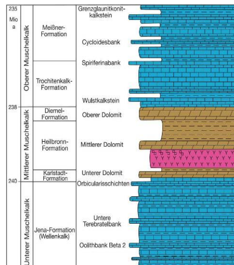
Abb. 1: Schemaprofil des Muschelkalks
