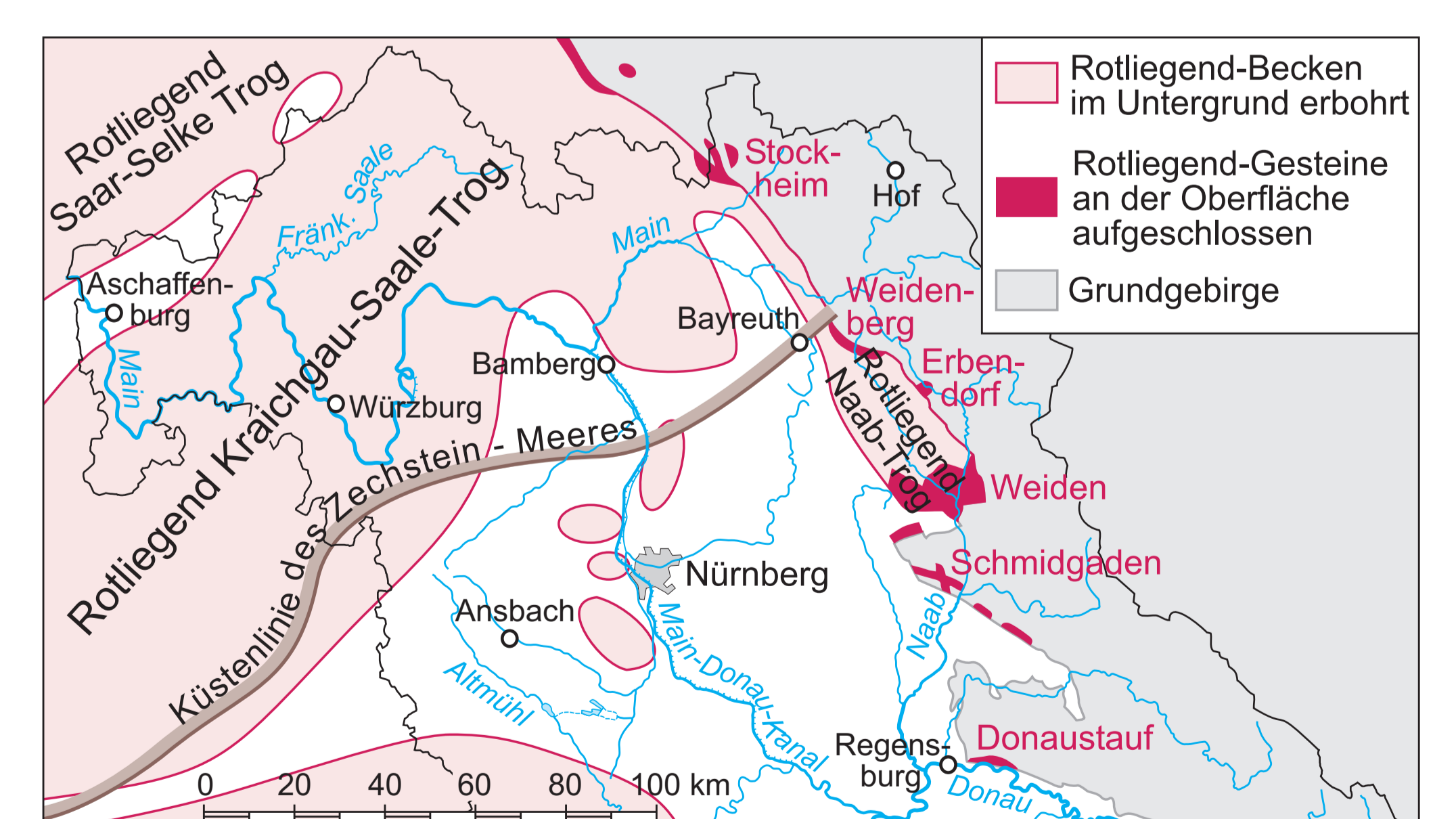
Verbreitung der Rotliegend-Becken und maximale Ausdehnung des Zechstein-Meeres in Nordbayern
