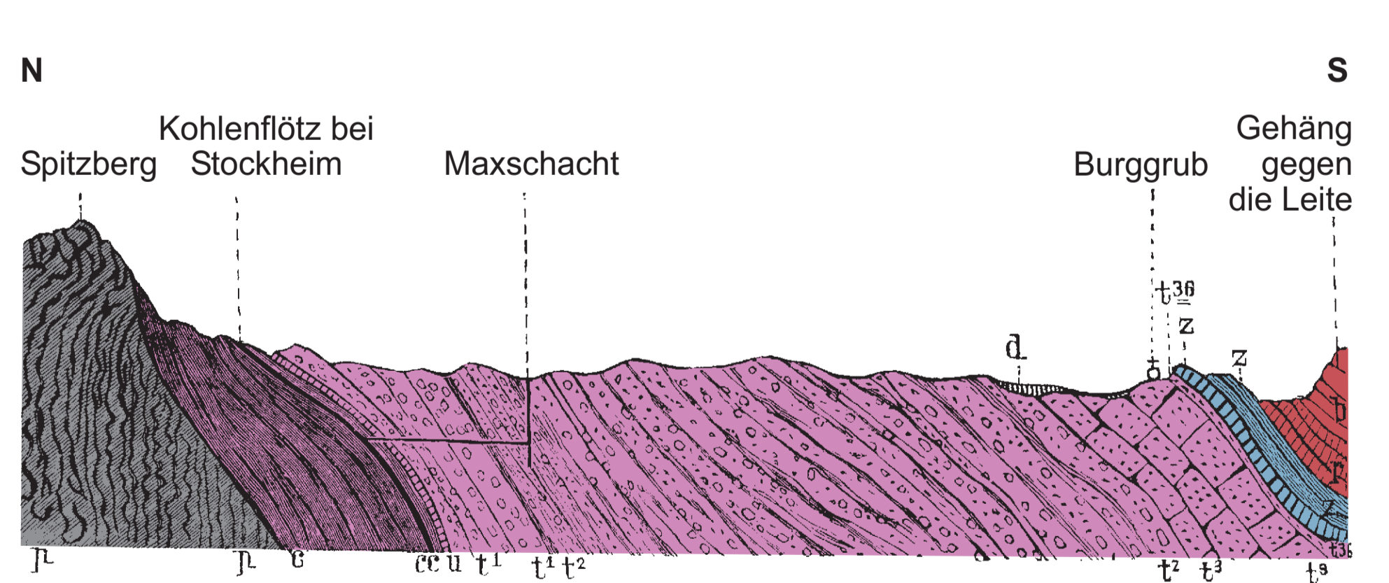
Geologisches Nord-Süd-Profil durch das Stockheimer Becken (Gümbel 1879) p-p: Kullmschichten; c: Carbonschichten; cc: Steinkohlenflöz; u: Übergangsschichten zu postcarbonischen Schichten; t 1 : unteres Rotliegendes; t 2 : mittleres Rotliegendes; t 3 : oberes Rotliegendes; t 4 : Weißliegendes und Kupferschiefer; z: Zechstein und rother Lettenschiefer; r: Leberschiefer des Buntsandsteins; b: unterer Buntsandstein
