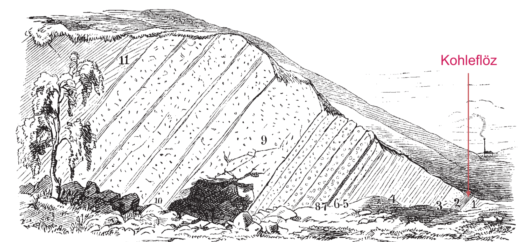
Hängende Schichten über dem Steinkohlenflöz im Steinbruch bei dem Catharinenschacht (Gümbel 1879) 2: Kohlenflöz 3-4: schwarze, unten sehr harte kieselige (3), oben weiche kohlige Schiefer-tone mit Pflanzeneinschlüssen; 5,2 m mächtig 5-6: grauer Kohlensandstein in Wechsellagerung mit grauem Schiefer-ton und einem Fischschuppen enthaltenden Brandschiefer-Flötzen; 1,0 m mächtig 7-8: 6-10 Bänke grauen Conglomerats, wechselnd mit grauem Sandstein und Schieferthon mit Pflanzenresten; 3,4 m mächtig 9: graue Conglomeratbänke von sehr großer Härte (als Strassenmaterial benutzt) und graue Thonig-sandige Schiefer-Zwischenlagen; 3,5 m mächtig 10-11: weniger mächtige Bänke rothen und grünlichen Conglomerats mit Zwischenlagen von grünlich-grauem sandigem Schiefer; 6,8 m mächtig
