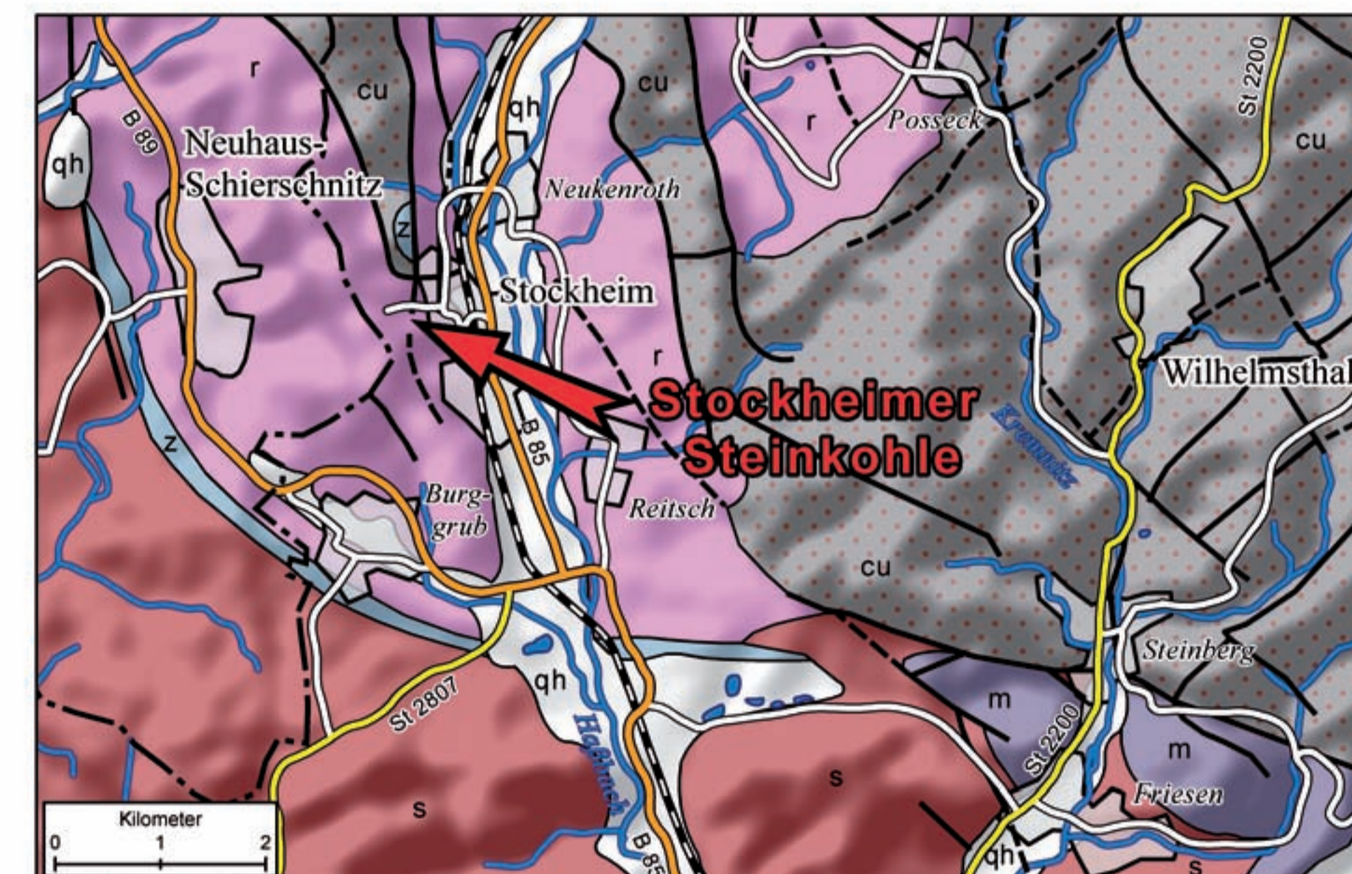
Geologische Karte der Umgebung von Stockheim Quartär: qh Talboden und jüngste Ablagerungen Trias: m Muschelkalk, s Buntsandstein Oberkarbon-Perm: z Zechstein, r Rotliegend Unterkarbon: cu Unterkarbon Siedlung über Geologie, Gewässer, Störung nachgewiesen / vermutet, Grenze Bayern-Thüringen
