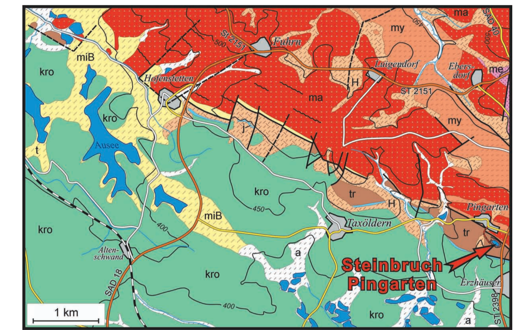
Geologische Karte der Umgebung von Pingarten
