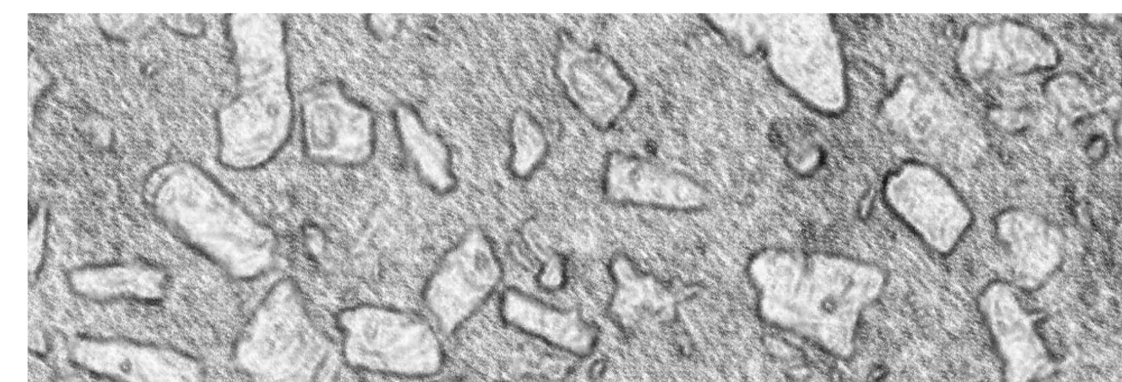
Porphyrisches Gefüge: Der Begriff „Porphyr“ wird streng genommen nur für magmatische – das heißt aus einer Schmelze entstandene – Gesteine verwendet. Die Einsprenglinge bestehen hier aus großen, in der Schmelze gewachsenen Einzelkristallen. Die Abbildung zeigt eine Dünnschliff-Fotografie eines magmatischen Gesteins mit porphyrischem Gefüge.
