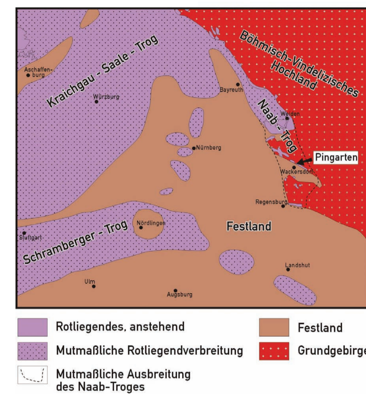
Verbreitung des Rotliegenden in Bayern
